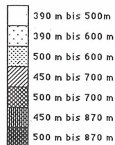
Abb. 4. Höhenumfang der einzelnen Flächen in der Stadt Zürich Altitudinal extent of the squares within the township of Zürich
