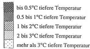
Abb. 2. Temperaturdifferenzen gegenüber den wärmsten Stellen in der Stadt Zürich, gemessen an einem klaren Sommerabend (nach SCHLATTER, verändert, aus LANDOLT 1991a) Temperature differences compared with the warmest localities in the township of Zürich on a clear summer evening (according to SCHLATTER, modified, from LANDOLT 1991a)
